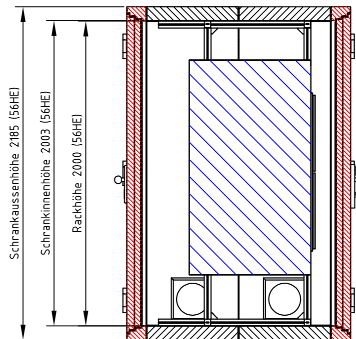
B-B ( 1 : 25 )
