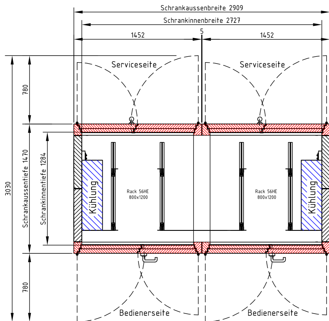
A-A ( 1 : 25 )
